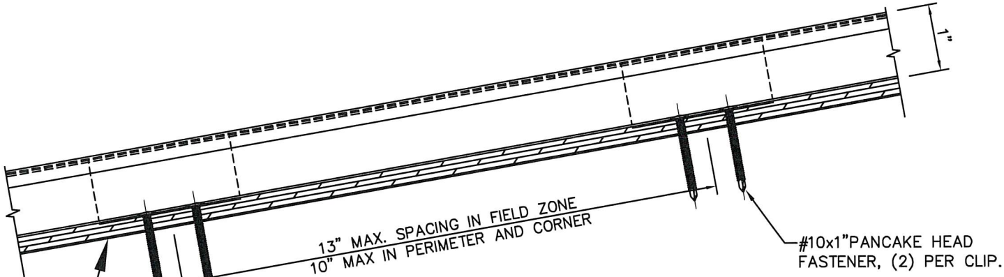
SECTION A-A
